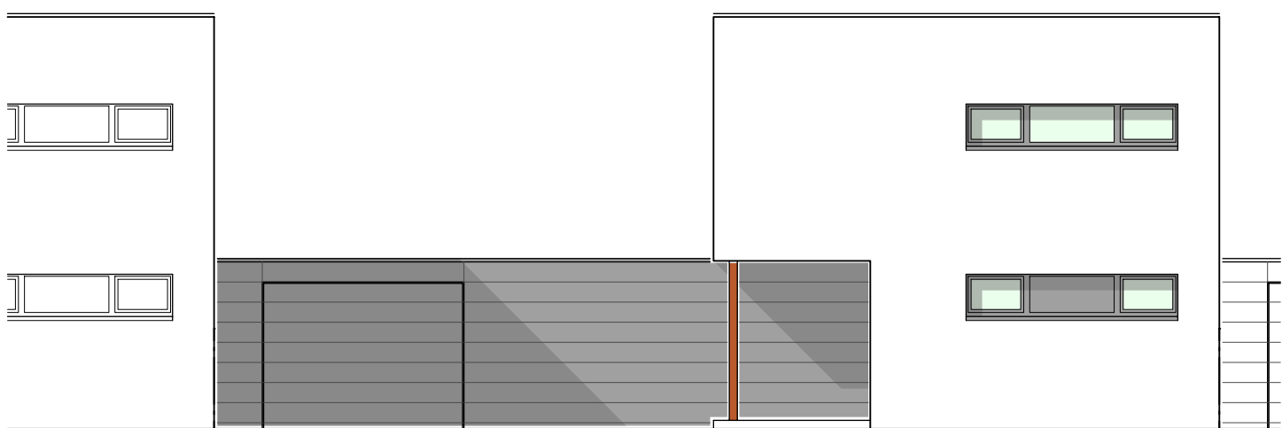
Ostansicht M 1:100
