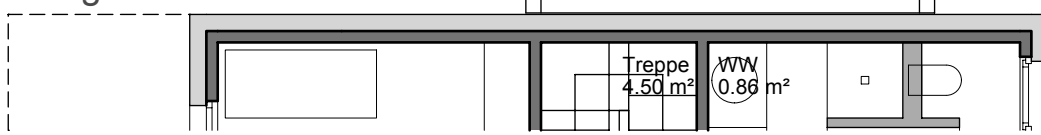
Grundriss Obergeschoss M 1:100
