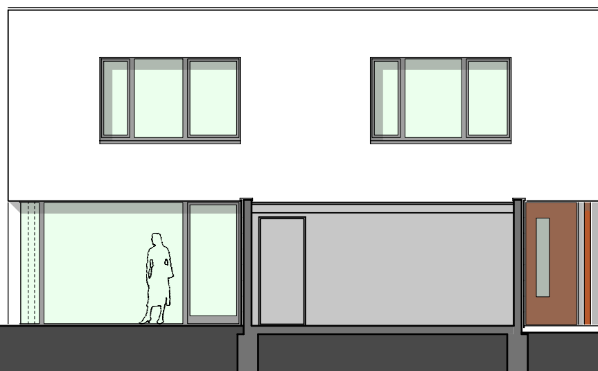
Südansicht M 1:100
